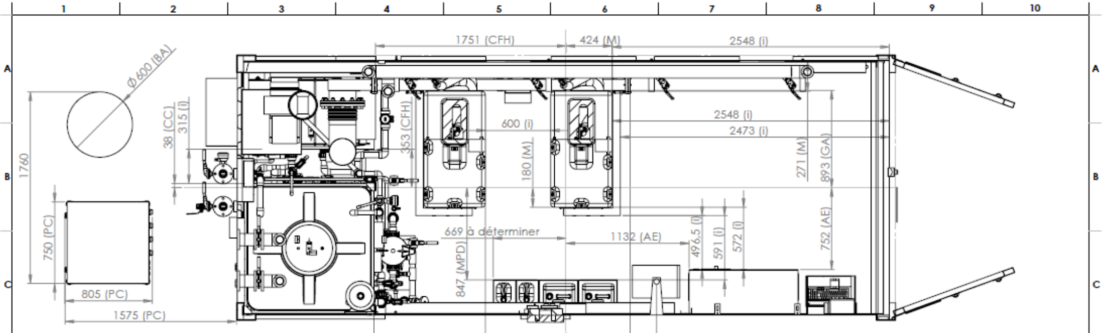
COUPE A-A Echelle 1 : 25
